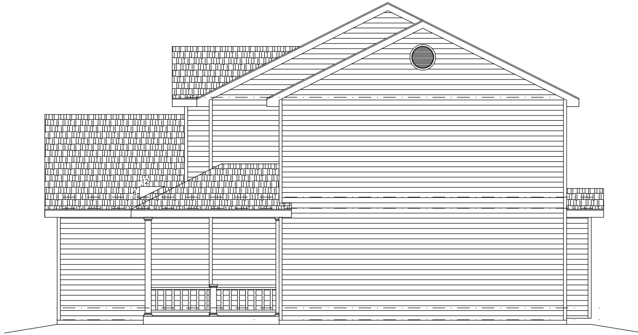
RIGHT ELEVATION
