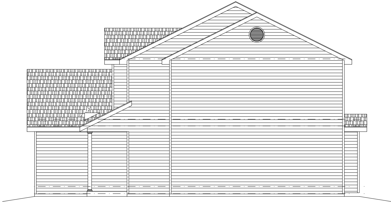
RIGHT ELEVATION
